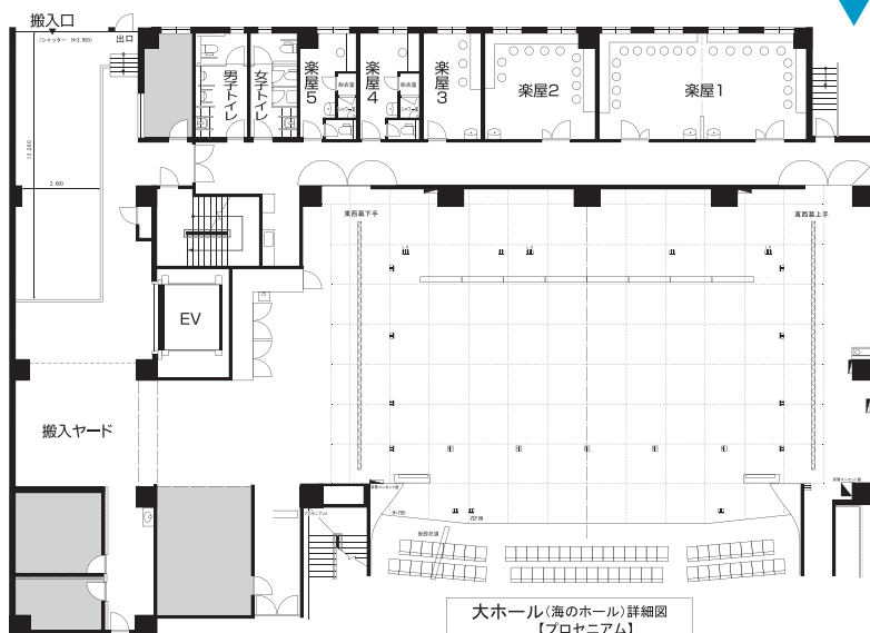
海のホール舞台図面
