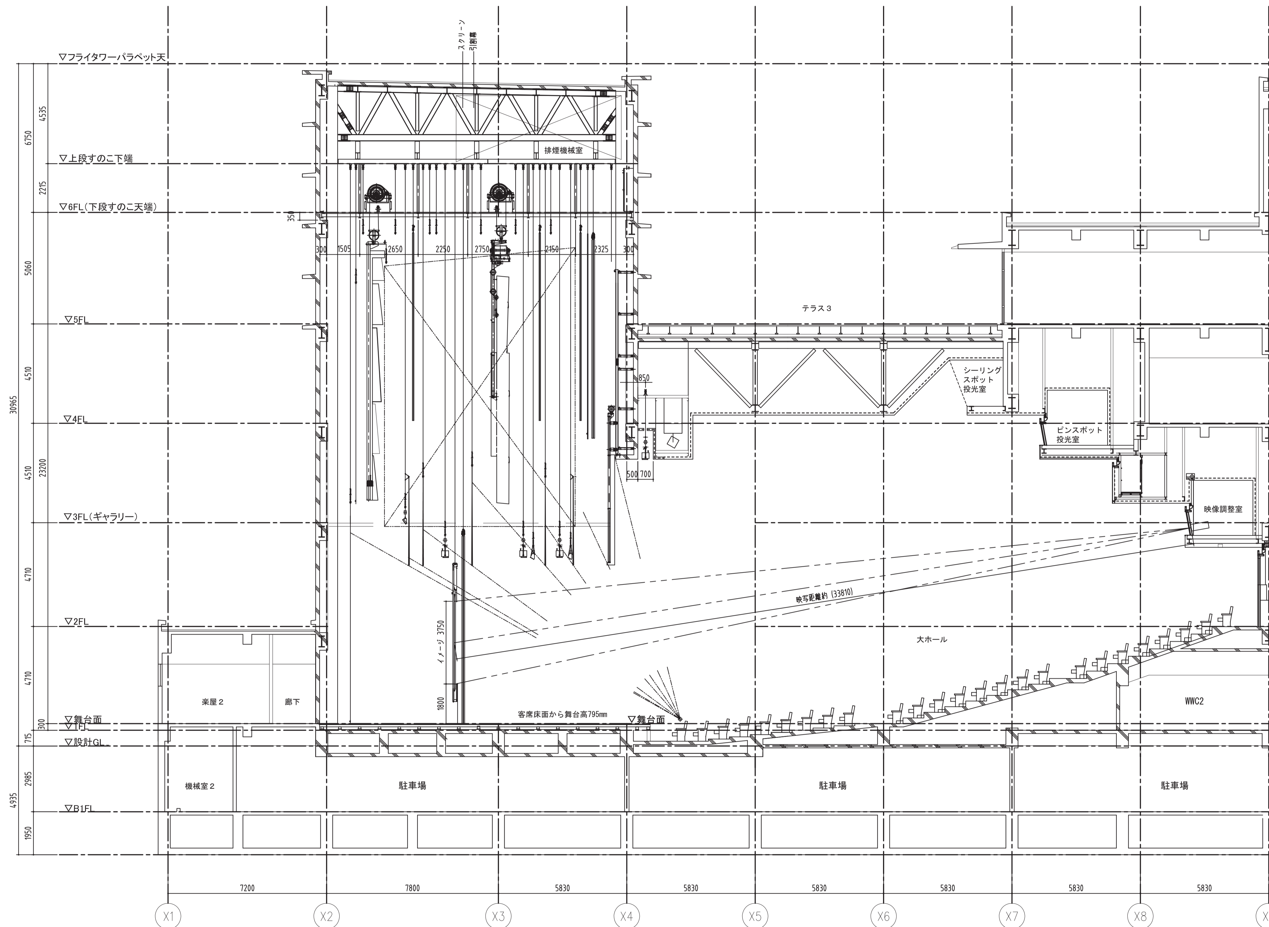
大ホール 断面図
